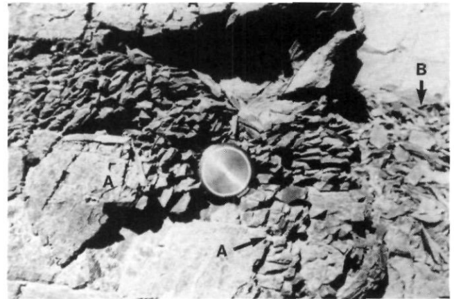
FIGURE 7. Intense fracturation des parois de schiste. A: réseau de fractures très serrées. B: concentration de plaquettes déjà détachées, en équilibre instable sur le dos d'une couche plus résistante.
