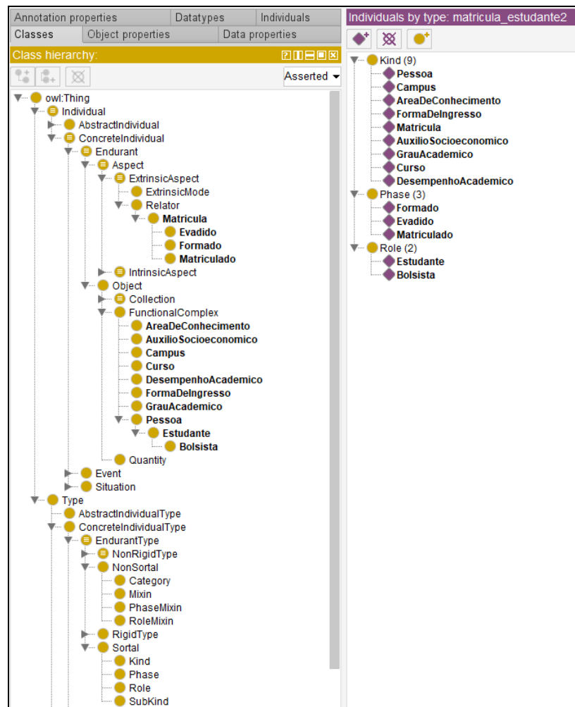
Figura 5: Integração das classes da Onto-Educacional com a UFO
