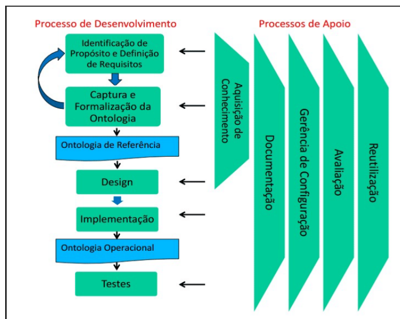
Figura 1: Processos e fases da Metodologia SABiO (adaptado e traduzido de [38]).
