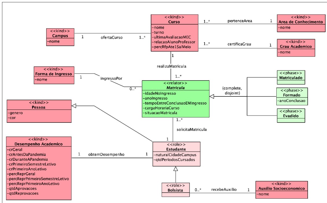
Figura 3: Ontologia de referência elaborada com OntoUML
