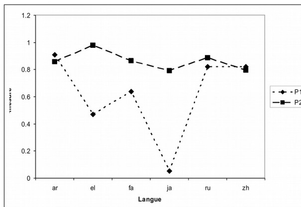
Figure 2.3 : Résultats d'Alinéa (système P2) pour la tâche d'alignement de corpus pré-segmenté.
