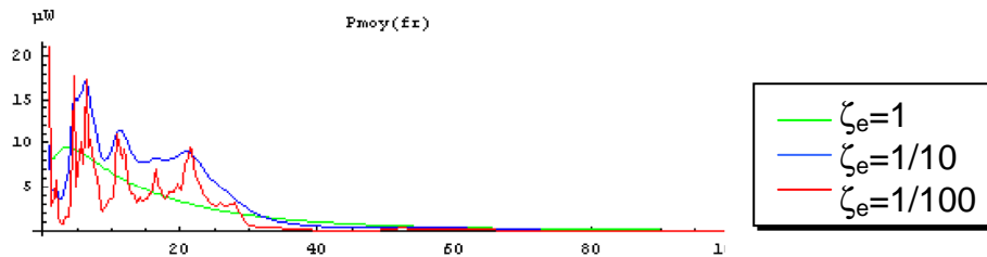
Figure 40 : Puissance récupérable sur une voiture à 50Km/h
