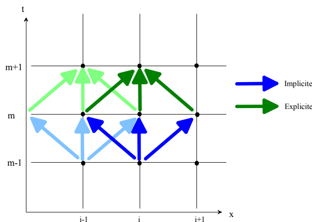
Figure 1 : Illustration des schémas implicite et explicite
