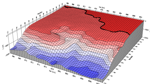
Figure 24 : Modèle numérique de la bathymétrie au large de Toulon (passage de 100m à 1500 de fond sur 8km)
