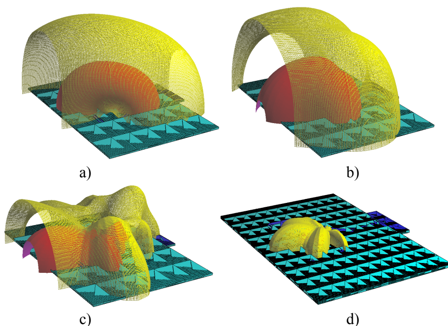
Figure 30 : Structure des champs lointains pour 1, 3, 5 et 9 GHz (a,b,c et d)
