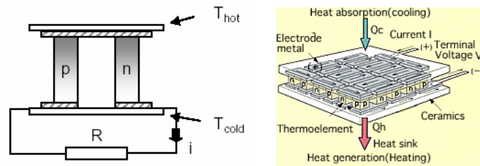
Figure 34 : Structures de composants thermoélectriques
