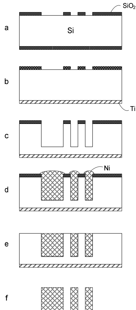
Figure 63 : Schéma de principe du process de réalisation de la nouvelle structure
